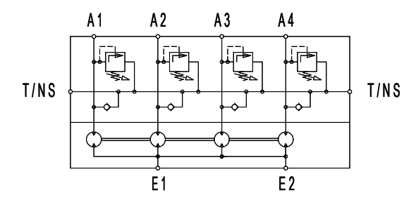
Sinnbild entsprechend DIN ISO 1219 circuit according DIN ISO 1219
